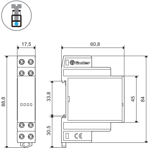
13.91 Винтовой зажим
