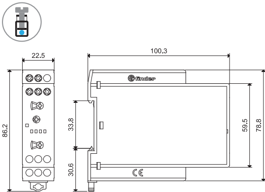
83.82 Винтовой зажим
