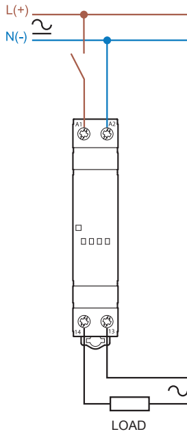
Однофазное подключение (77.01)
