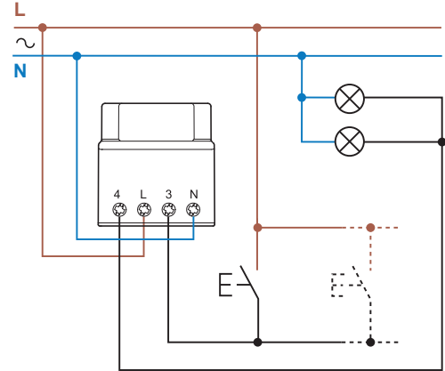
Тип 15.91 - 4-проводное соединение
