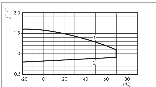
R 67 - Отношение рабочего диапазона к температуре окр. среды, 67.xx-4300 при стандартном питании катушки (-40...+70)°C
