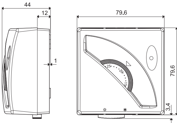
Габаритный чертеж
