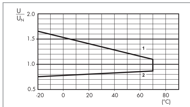
R 48 - Отношение рабочего диапазона для AC к температуре окр. среды
