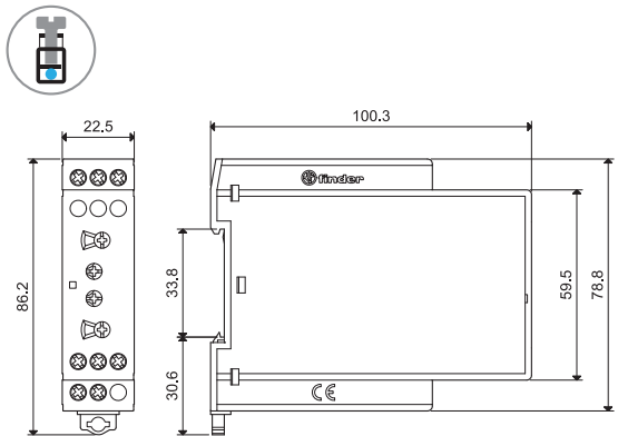
83.91 Винтовой зажим
