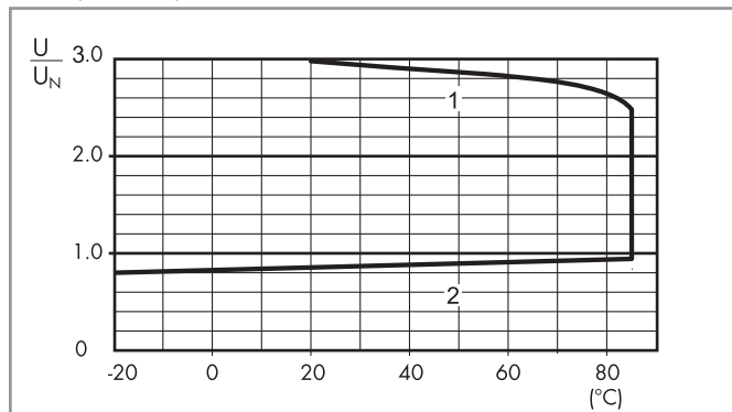
R 67 - Отношение рабочего диапазона к температуре окр. среды, 67.xx-4500 при энергосберегающем режиме питания катушки (-40...+85)°C
