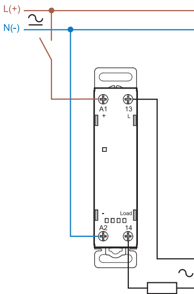
Однофазное подключение (77.31.....7x)
