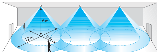
Групповая установка
