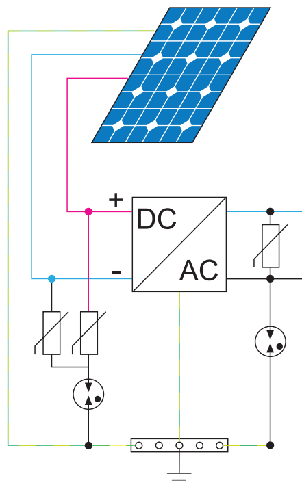
Рис 10: пример фотогальванической системы для здания не оборудованного системой защиты от молнии; защита со стороны DC при помощи SPD с U_{oc\ stc} = 420\text{ В} , и защита со стороны AC устройством 7P.22, характерным для систем TT.
