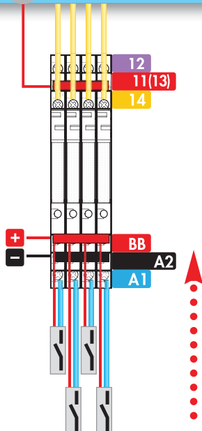
Входные устройства
