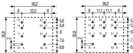
62.22 Вид сбоку
