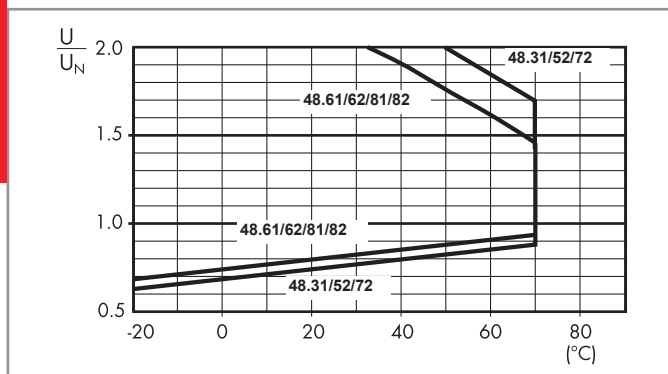
R 48 - Отношение рабочего диапазона для DC к температуре окр. среды
