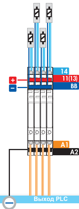
Выходные устройства
