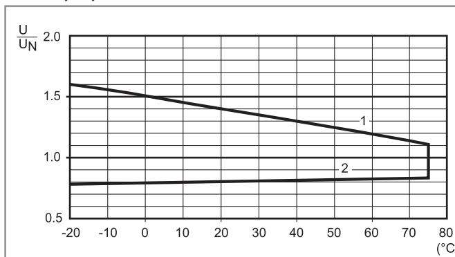
Р 65 - Отношение рабочего диапазона для AC к температуре окр. среды
