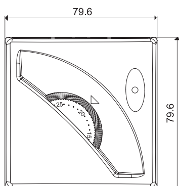
Габаритный чертеж
