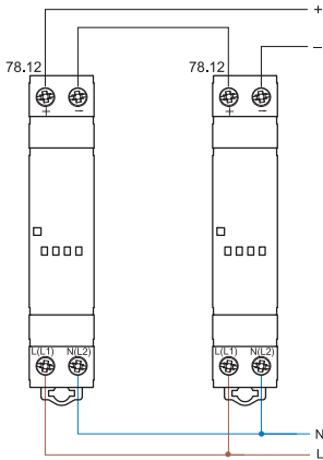
последовательное соединение
