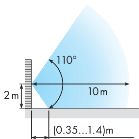
18.01, 18.11 - Настенный монтаж
