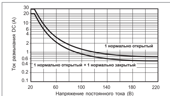
Н 65 - Макс. отключающая способность DC1
