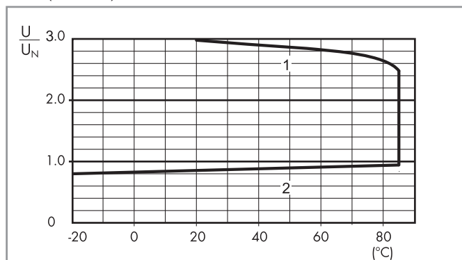
R 67 - Отношение рабочего диапазона к температуре окр. среды, 67.xx-4300 при энергосберегающем режиме питания катушки (-40...+85)°C
