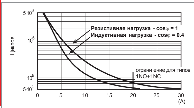
Ф 65 - Электрическая долговечность (AC) при ном. нагрузке
