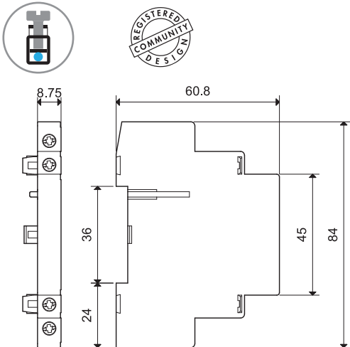
Тип 022.33 / 022.35 Винтовой зажим
