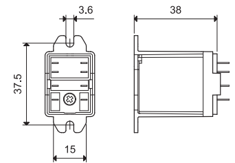
056.25 с реле
