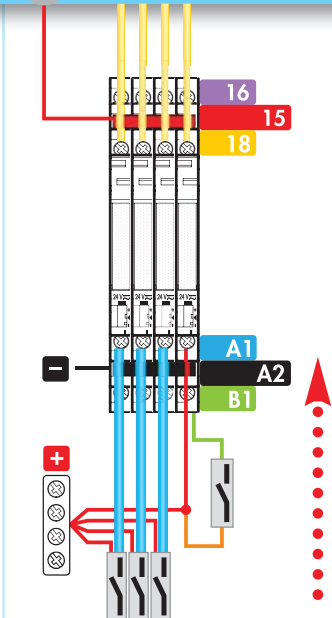
Входные устройства
