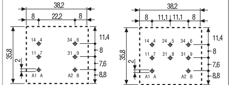
62.22 - 0300 Вид сбоку
