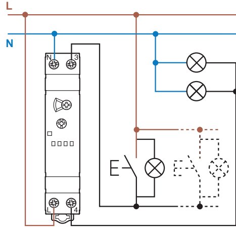
4-проводное соединение
