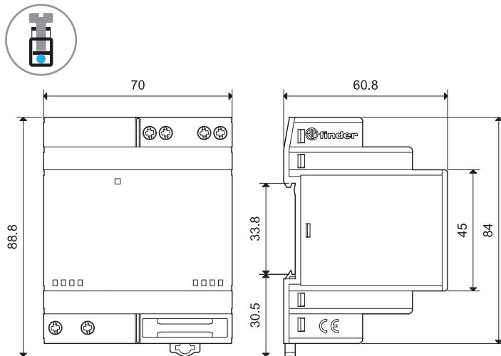
78.36 Винтовой зажим
