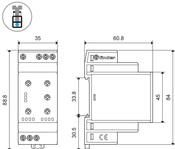
70.41 Винтовой зажим
