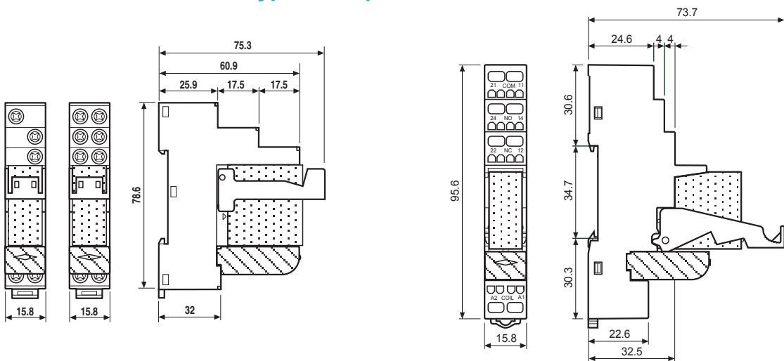
48.31 48.52 / 48.61 / 48.62 Винтовой зажим
