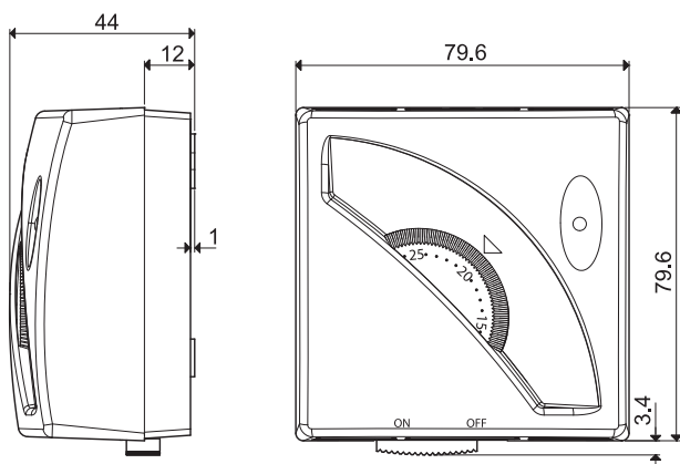
Габаритный чертёж
