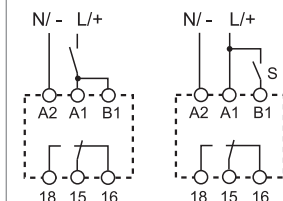
Схема подключения (без сигнала START)
