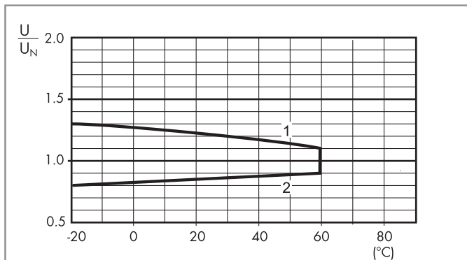
R 67 - Отношение рабочего диапазона к температуре окр. среды, 67.xx-4500 при стандартном питании катушки (-40...+60)°C
