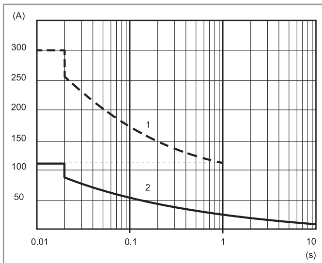
L77-3 Зависимость пикового пускового тока (AC) от времени 77.01.х.ххх.80хх
