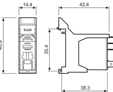
046.07 с реле
