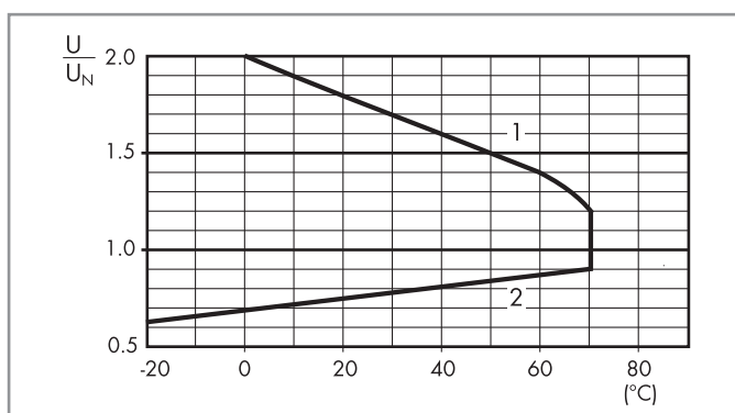
R 48 - Отношение рабочего диапазона для DC к температуре окр. среды - типы 48.12
