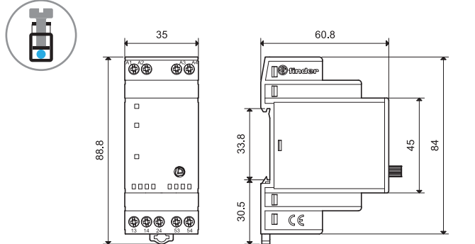
Тип 19.42 Винтовые клеммы
