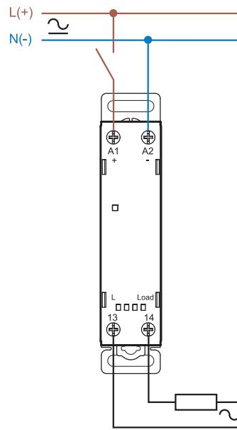
Однофазное подключение (77.31.....5x)
