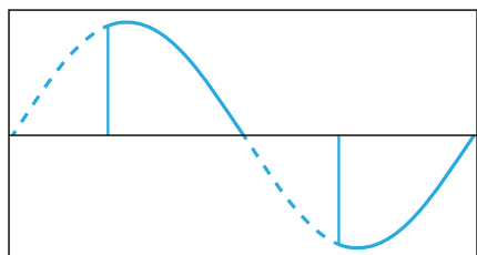
Диммирование по переднему фронту
