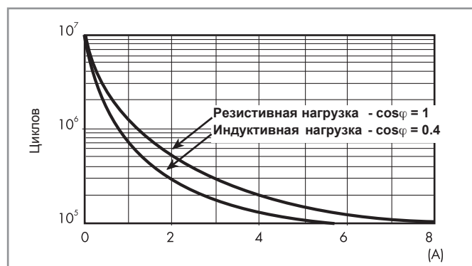
F 48 - Электрическая долговечность (АС) при ном. нагрузке, Типы 48.12
