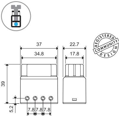
13.91 Винтовой зажим
