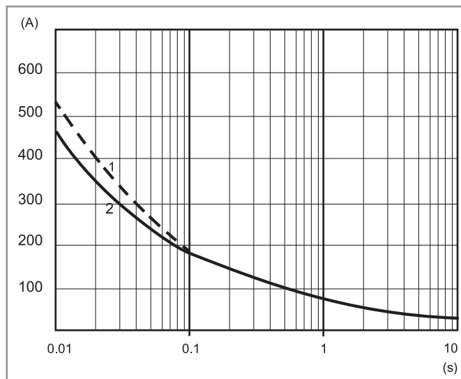
L77-5 Зависимость пикового пускового тока (AC) от времени 77.31.х.ххх.80хх
