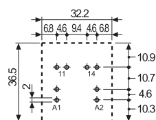
Вид сбоку
