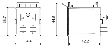
065.08 с реле
