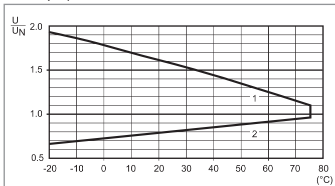
Р 65 - Отношение рабочего диапазона для DC к температуре окр. среды
