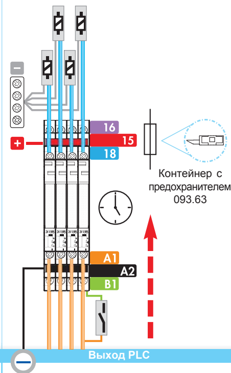
Выходные устройства
