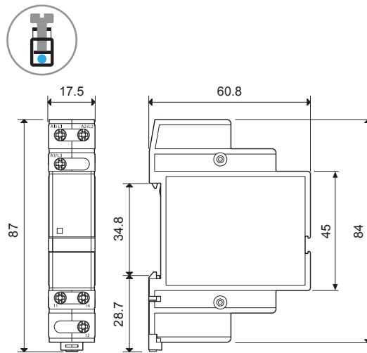
70.61 Винтовой зажим
